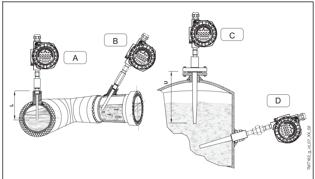
Fig. 3: Exemples d'installation
