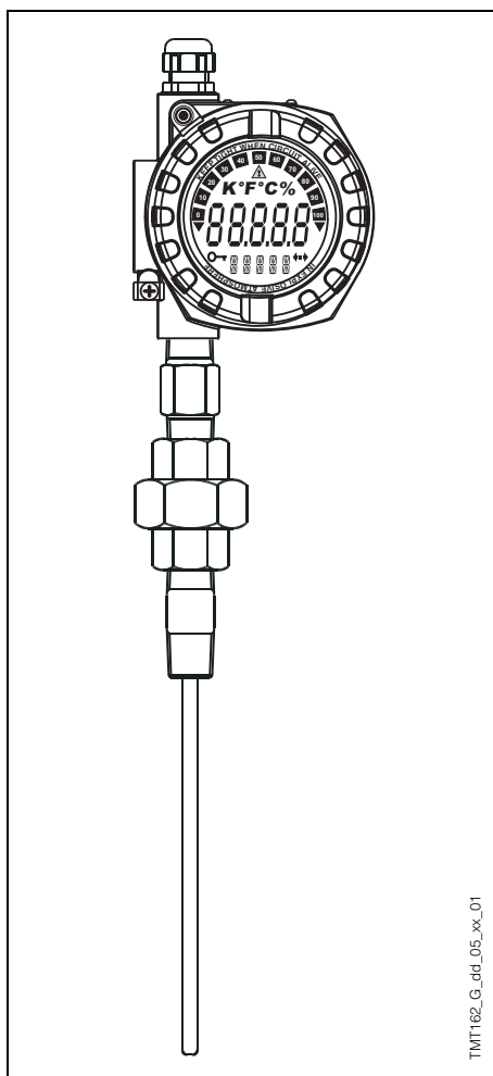
Fig. 1: TMT 162R avec les différents types d'extension
