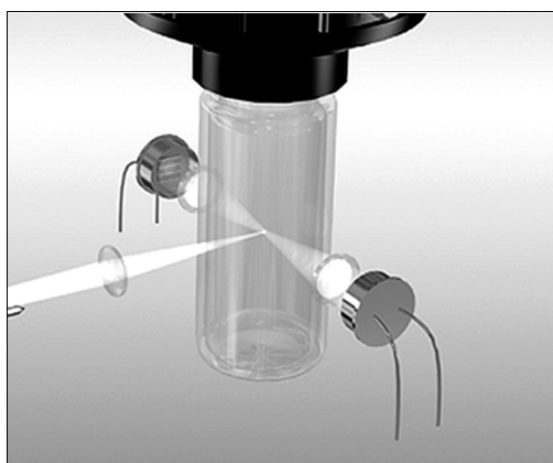
Méthode de la lumière diffusée à 90°
