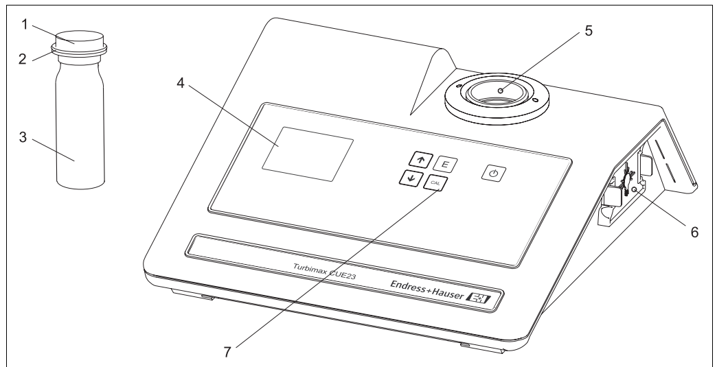
Ensemble de mesure Turbimax CUE23 (exemple)
