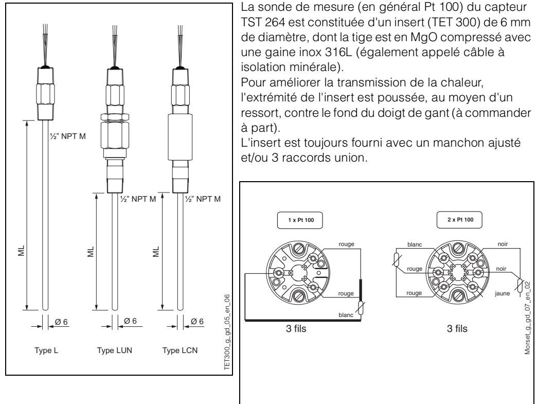
Fig. 6 : Sonde, dimensions et câblage interne
