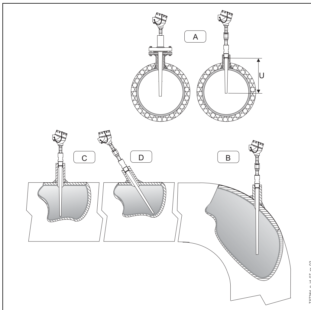
Fig. 2 : Montage sur conduite ou cuve au moyen de raccords filetés ou à bride
