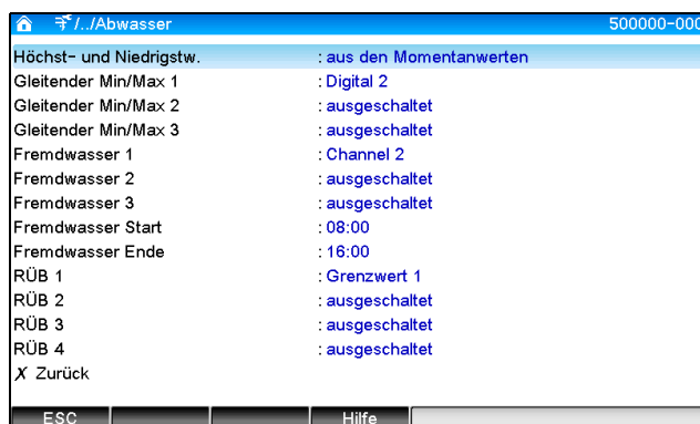
Abb. 3: Applikation - Abwasser
