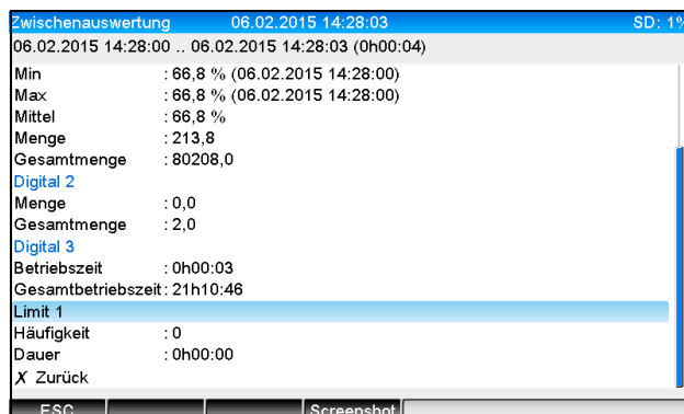
Abb. 7: Signalauswertung mit Alarmstatistik
