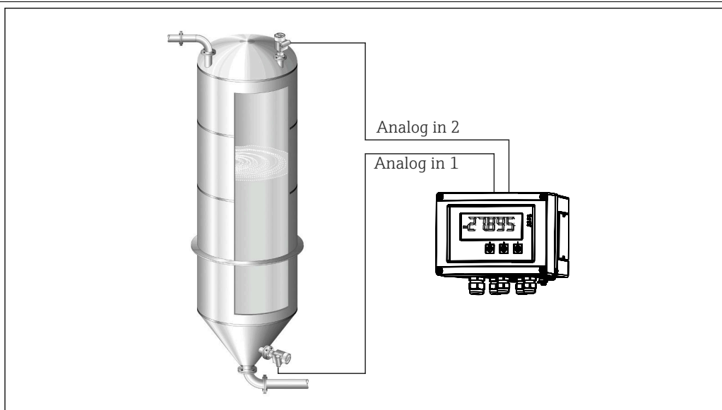
Fig. 1 Ejemplo para una aplicación de "presión diferencial"
