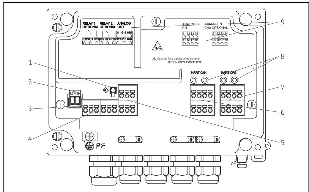
2 Vista interior y asignación de terminales del indicador de proceso
