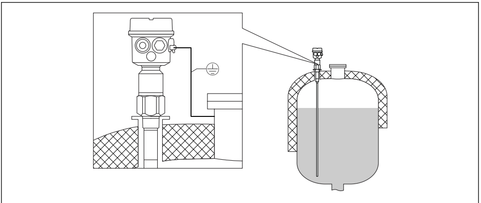
3 Sonde avec longueur inactive pour cuves isolées
