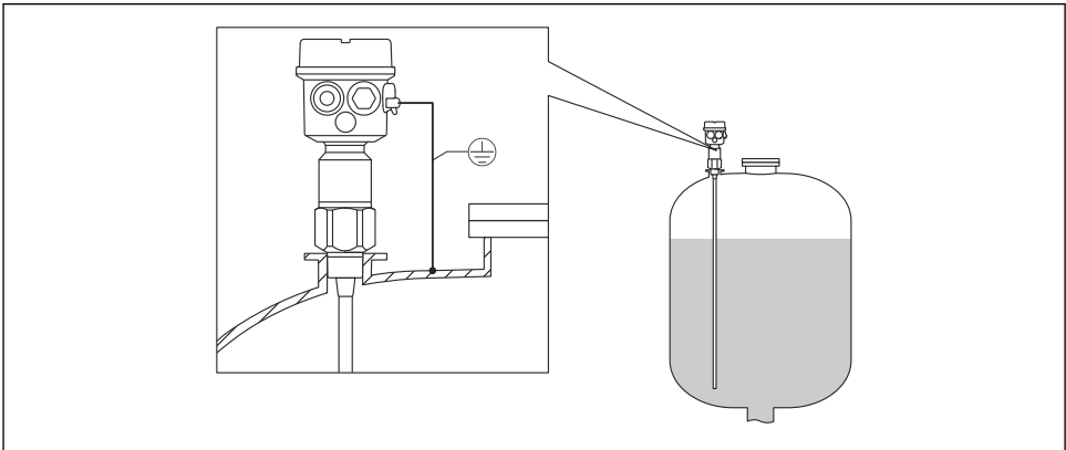
1 Sonde avec cuves conductrices
