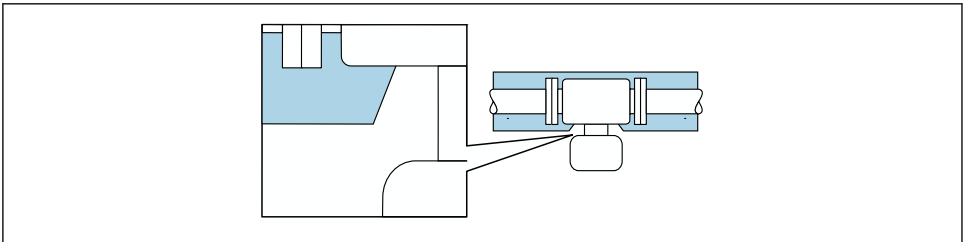
12 Isolation thermique avec tube prolongateur non isolé
