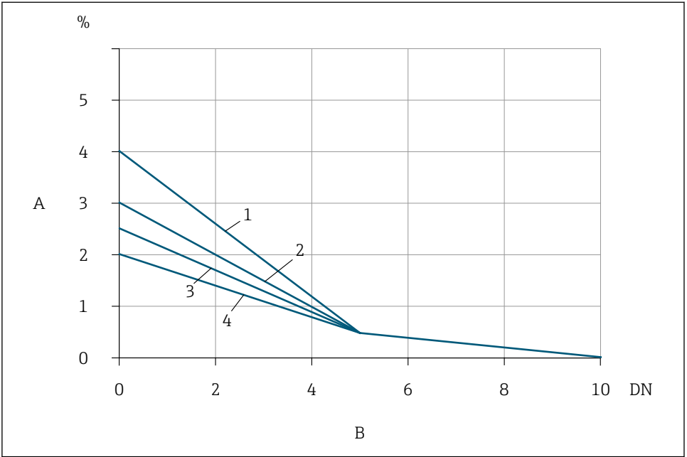
10 Écart de mesure supplémentaire auquel il faut s'attendre avec les tranquillisateurs de débit en fonction du type de perturbation et de la longueur droite d'entrée
