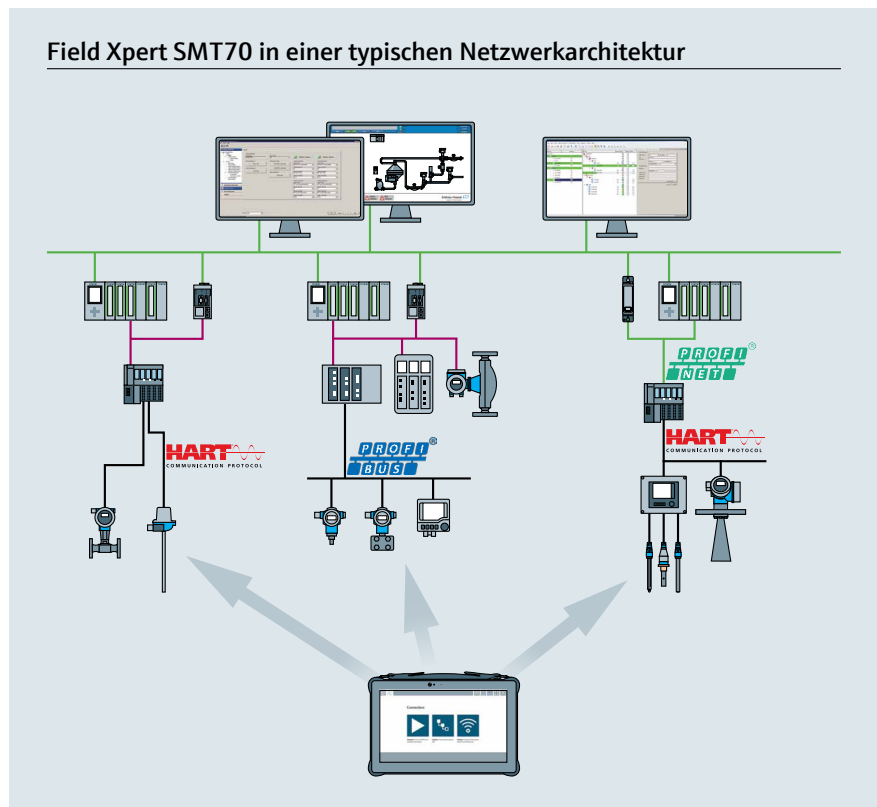
Field Xpert SMT70 als mobiler Arbeitsplatz direkt im Feld
