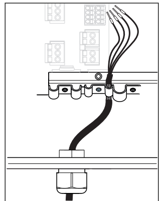
20 Schraube festziehen (2 Nm (1,5 lbf ft))
