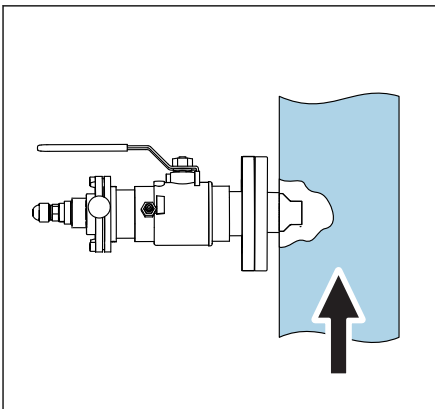
14 Einbau mit Wechselarmatur CUA451
