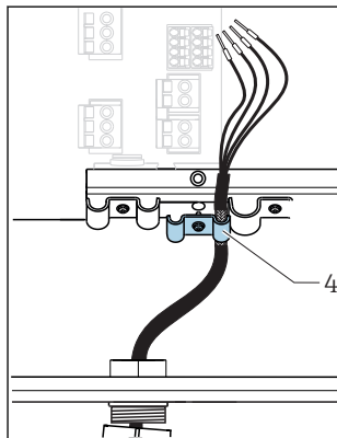
19 Kabel einlegen
