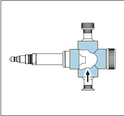
13 Einbau mit Durchflussarmatur CYA251
