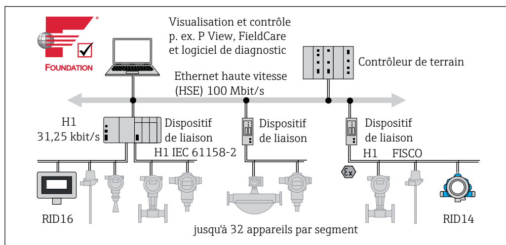
1 Intégration système via FOUNDATION Fieldbus™
