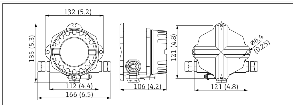
4 Dimensions de l'afficheur de terrain ; dimensions en mm (in)
