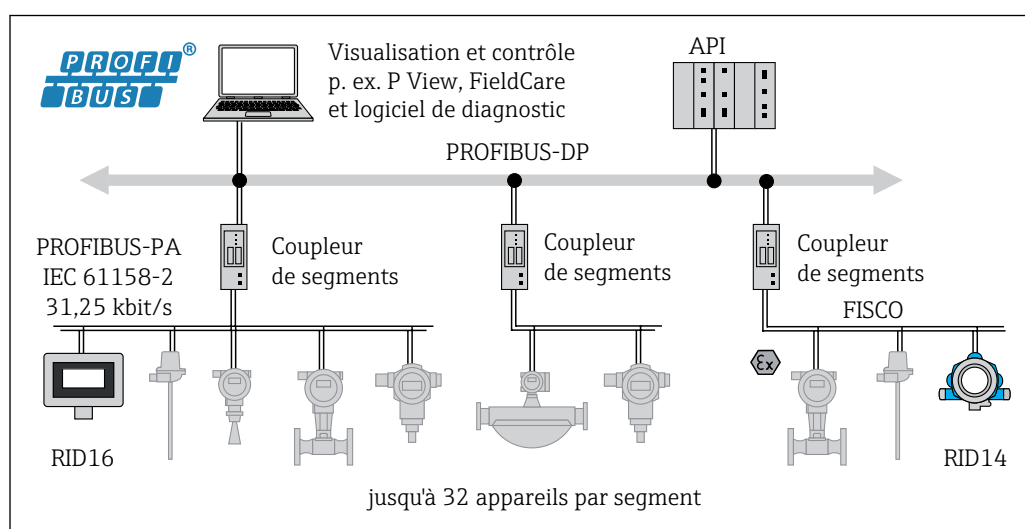
2 Intégration système via PROFIBUS® PA
