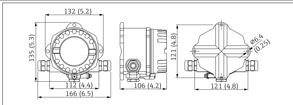
4 Dimensiones del indicador de campo; dimensiones en mm (pulgadas)
