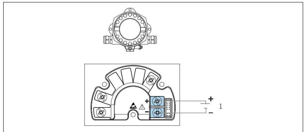
3 Asignación de terminales del indicador de campo
