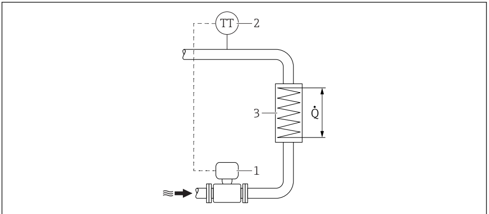
3 Disposición para medidas de diferencias delta de temperatura en vapor saturado o en agua
