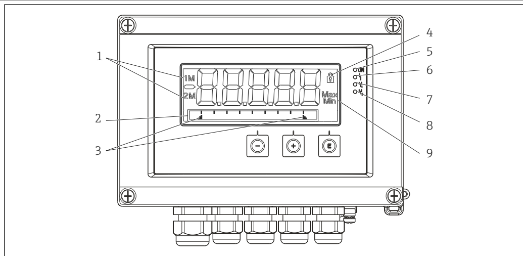
4 Affichage de l'afficheur de terrain
