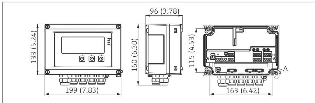
3 Dimensions de l'afficheur de terrain en mm (in)
