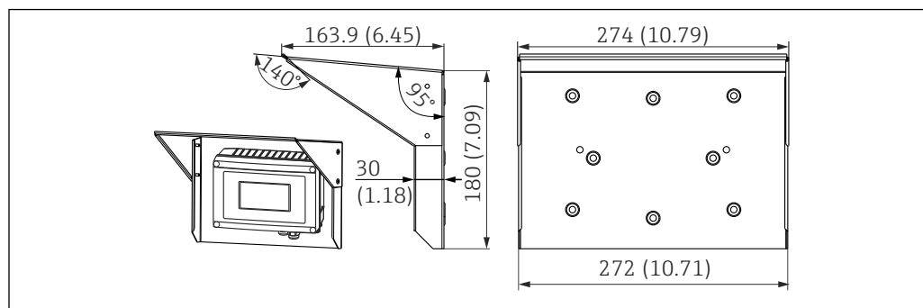
5 Dimensions en mm (in)
