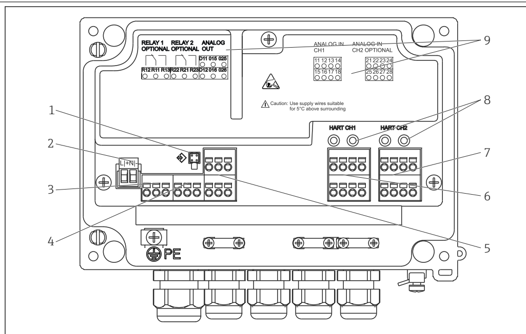
2 Vue de l'intérieur et affectation des bornes de l'afficheur de process
