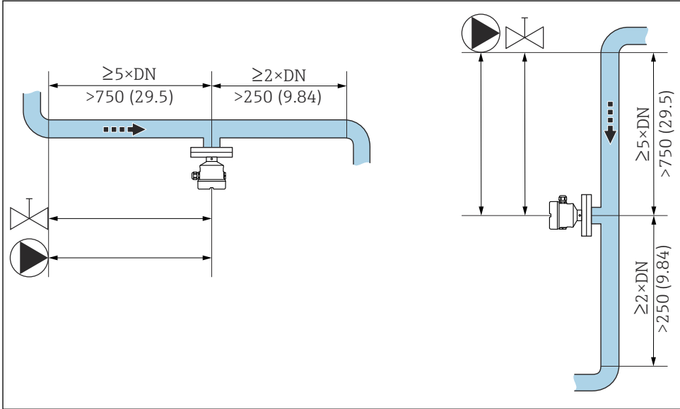
4 Montage de la section d'entrée. Unité de mesure mm (in)
