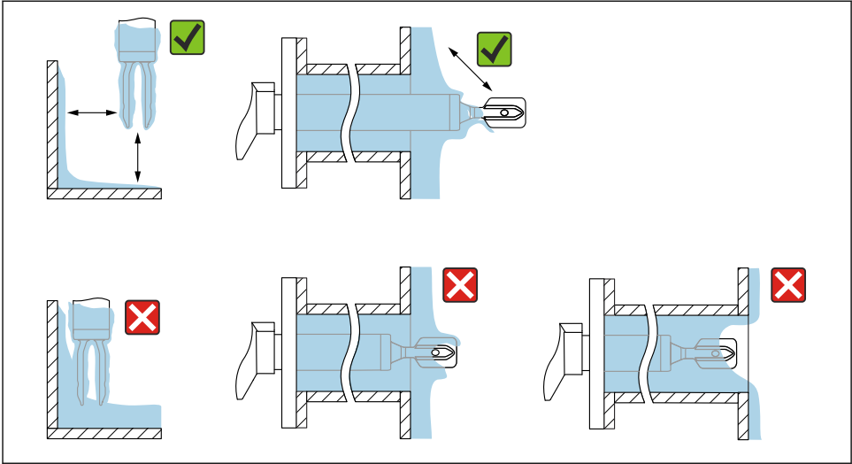
6 Installasjonseksempler for et svært viskøst prosessmedium
