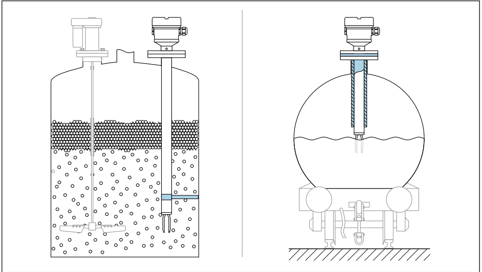
8 Eksempler på støtte ved dynamisk last
