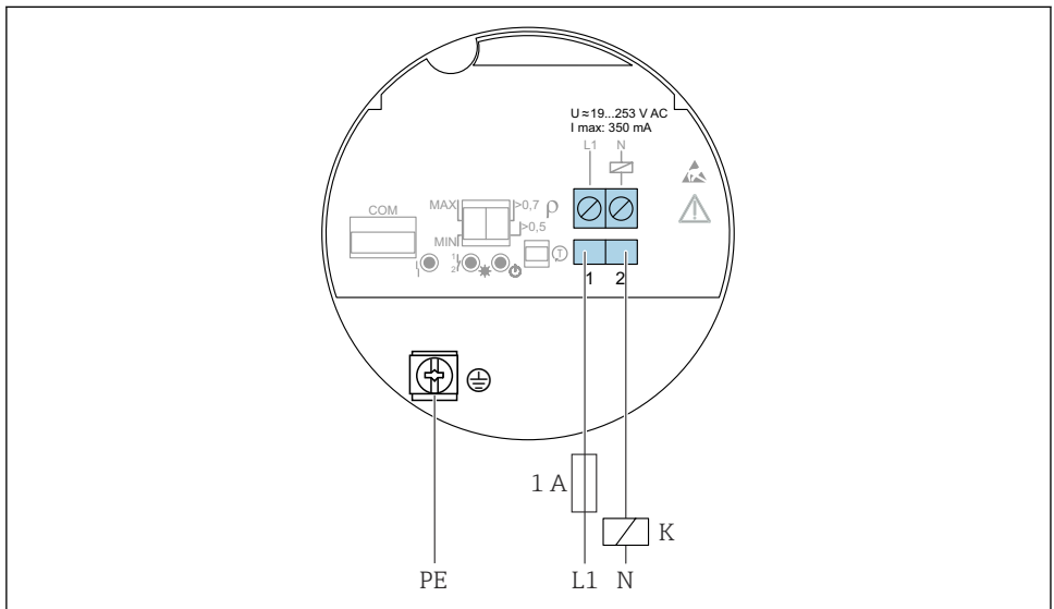
13 2-tråds AC, elektronikkinnsetts FEL61
