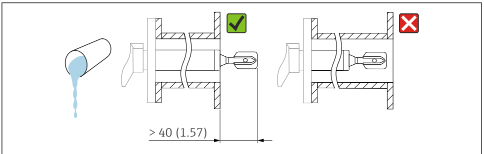
7 Installatievoorbeeld voor een vloeistof met hoge viscositeit. Maateenheid mm (in)
