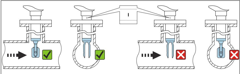
12 Installatie in leidingen (houd rekening met vorkpositie en markering)
