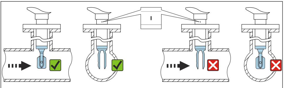
12 Instalación en tuberías (tenga en cuenta la posición de la horquilla y las marcas)
