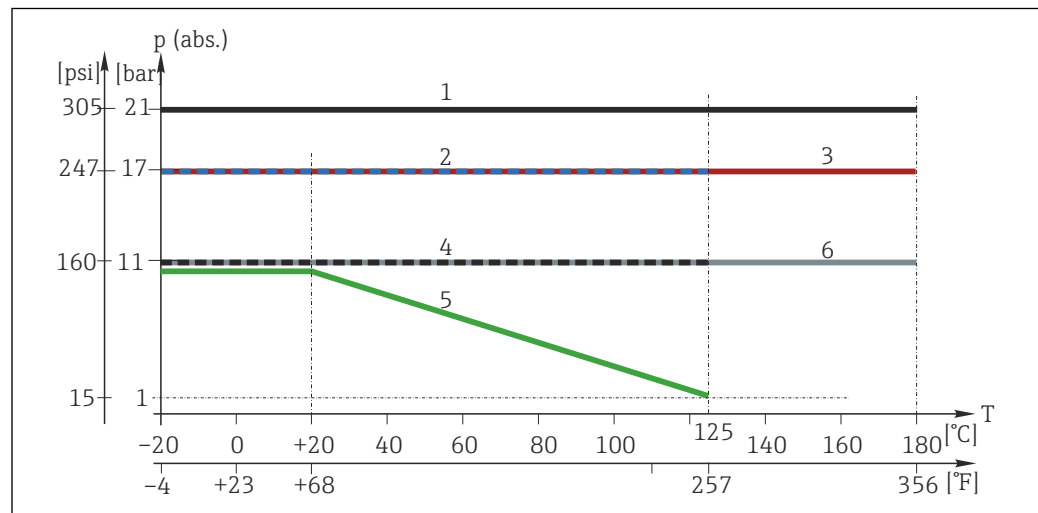
12 Druck-Temperatur-Kurven
