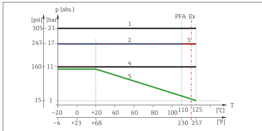
11 Druck-Temperatur-Kurven
