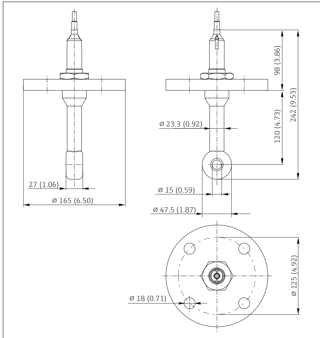
■ 15 Ausführung Flansch EN1092-1 DN50 PN16, 316L verschweißt PFA-Dichtplatte Sensor. Maßseinheit mm (in)
