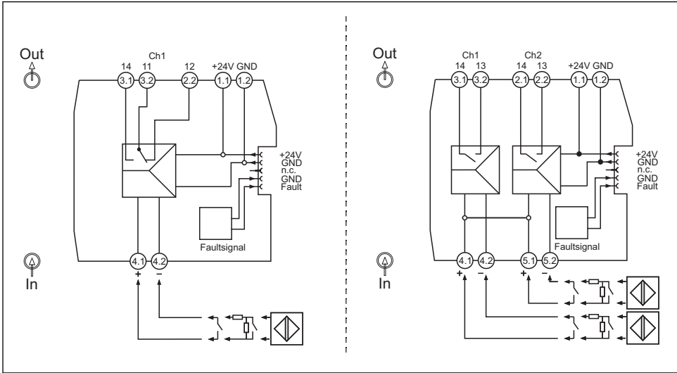
4 Affectation des bornes du RLN22 : version à 1 voie (à gauche), version à 2 voies (à droite)
