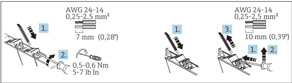
3 Raccordement électrique à l'aide des bornes à vis (à gauche) et des bornes enfichables (à droite)
