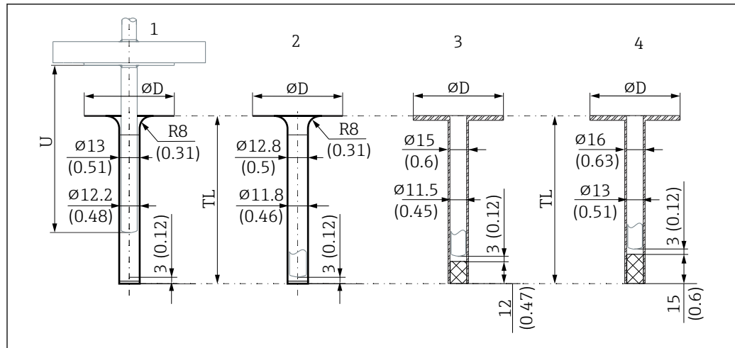
图 1 外护套的外形尺寸示意图；单位：mm (in)。不同材质的外护套的尺寸参数存在差异。
