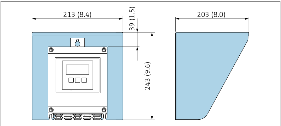
14 Wetterschutzhaube Proline 500; Maßeinheit mm (in)
