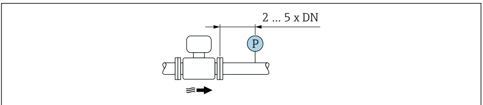
11 Einbau einer Druckmessstelle (P = Drucktransmitter)
