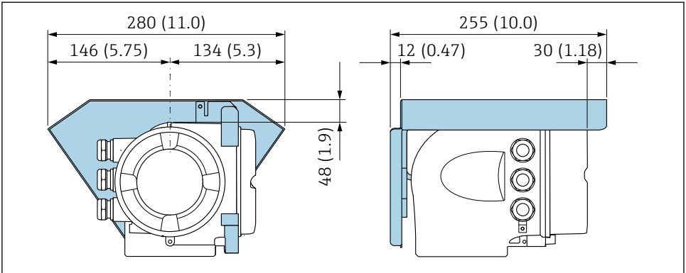
13 Maßeinheit mm (in)
