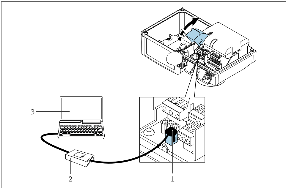
2 Anschluss Laptop via Commubox FXA291 an der Serviceschnittstelle
